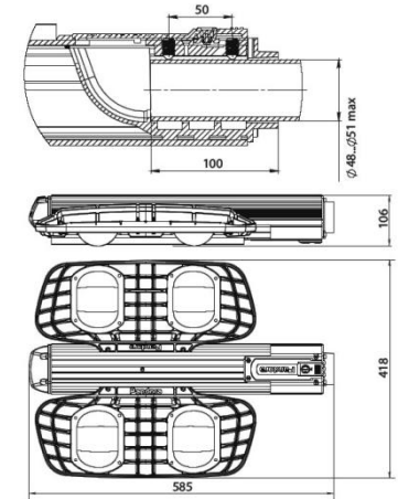
Рисунок 3. Габаритный чертеж
